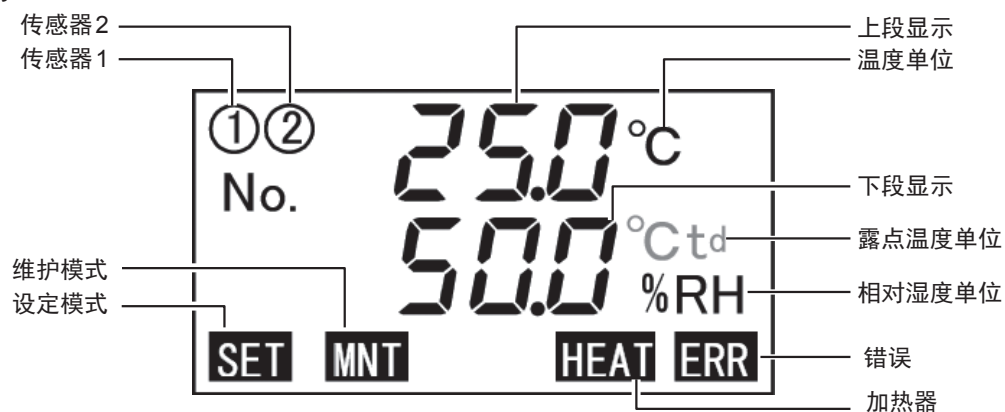
图 30 LCD 显示
