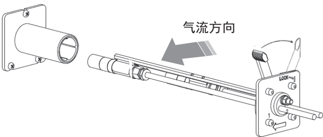
图 11 气流方向
