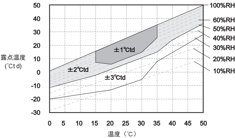
图 3 室内用 露点温度精度
