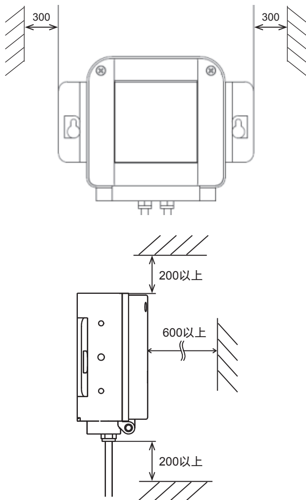
图 12 维修空间
