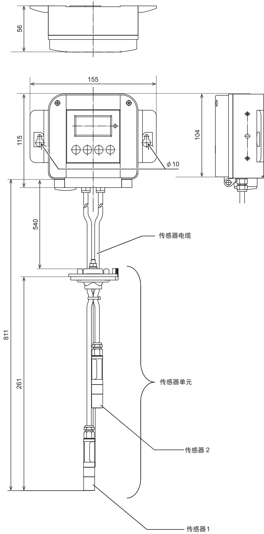
图 6 风管安装类型 外形尺寸图 (mm)
