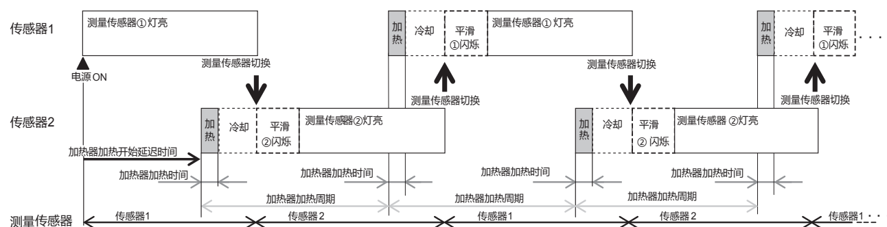
图29 电源ON后的基本动作 (传感器1从测量传感器开始的情况)
