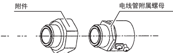
图 24 电线管连接头
