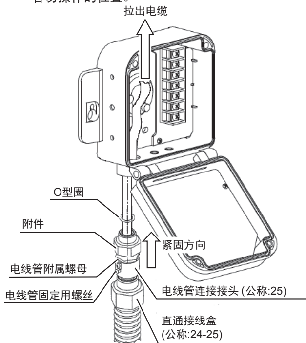
图 25 电线管安装
