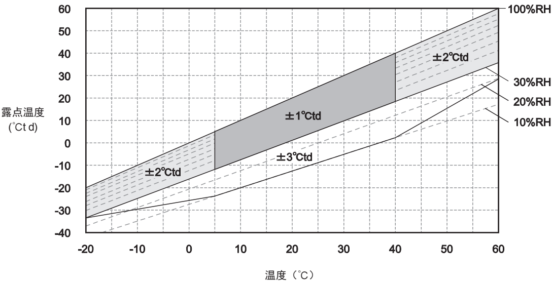
图 4 风管用 露点温度精度 (外壳环境温度 25°C)
