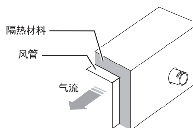
图 19 隔热材料的施工
