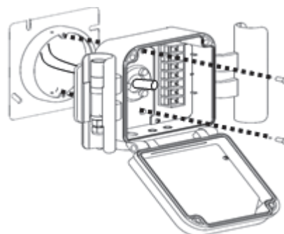
图 15 外壳的安装
