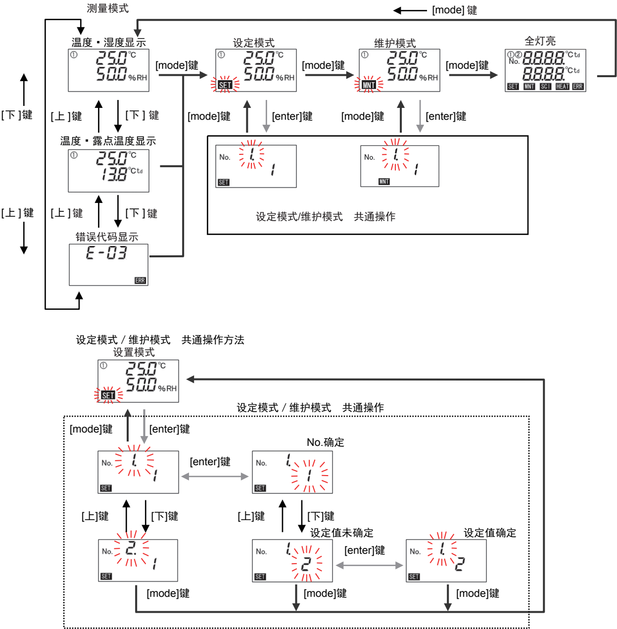
图 31 操作模式关联图（设定模式的场合）
