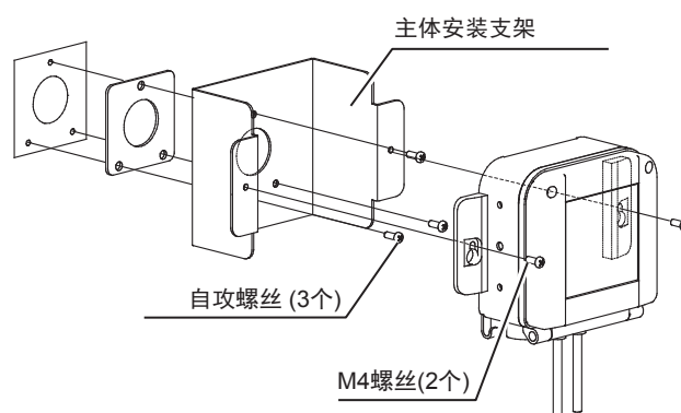
图 20 外壳的安装
