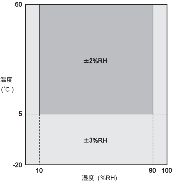
图 2 风管用 湿度精度
