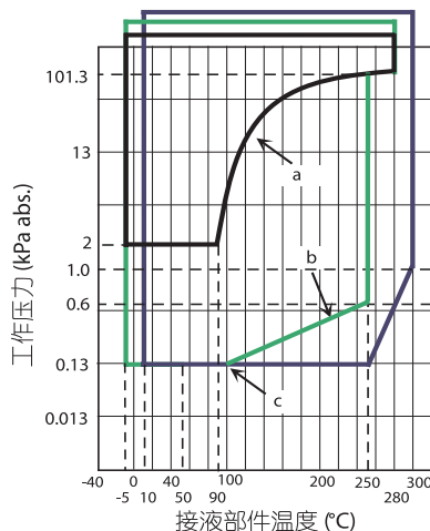
图 4 接液部工作压力及温度 (高温型/ 高温真空型 / 高温高真空型)
