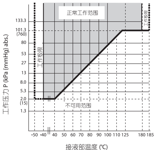
图 1 接液部工作压力及温度 (普通型)
