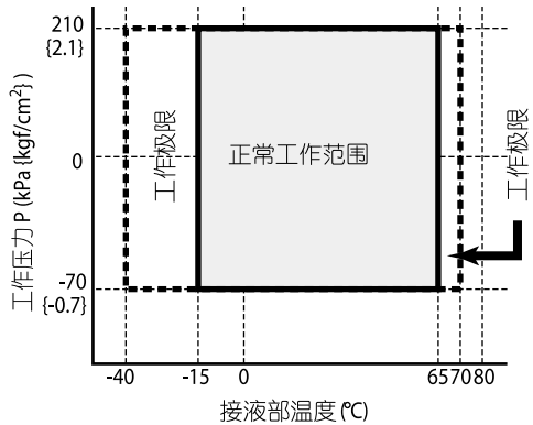
图 3 接液部工作压力及温度 (GTX15D 型普通型)
