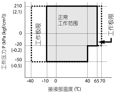
图 4 接液部工作压力及温度 (GTX15D 型氧用)
