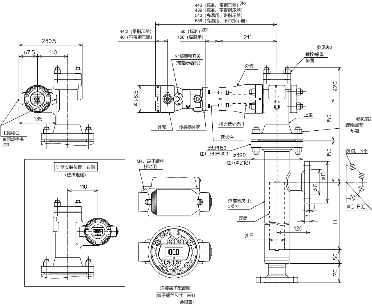
S-B: 侧面 - 底部 [单位 : mm]
