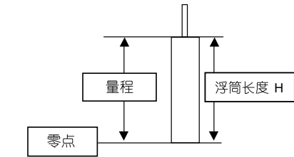
图 7 调整的正确方式： 将浮筒底部设置在零点
