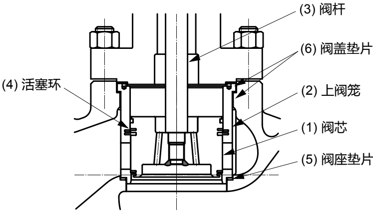
图 4. 阀内件结构图 ( 伸长 1 型阀盖 )
