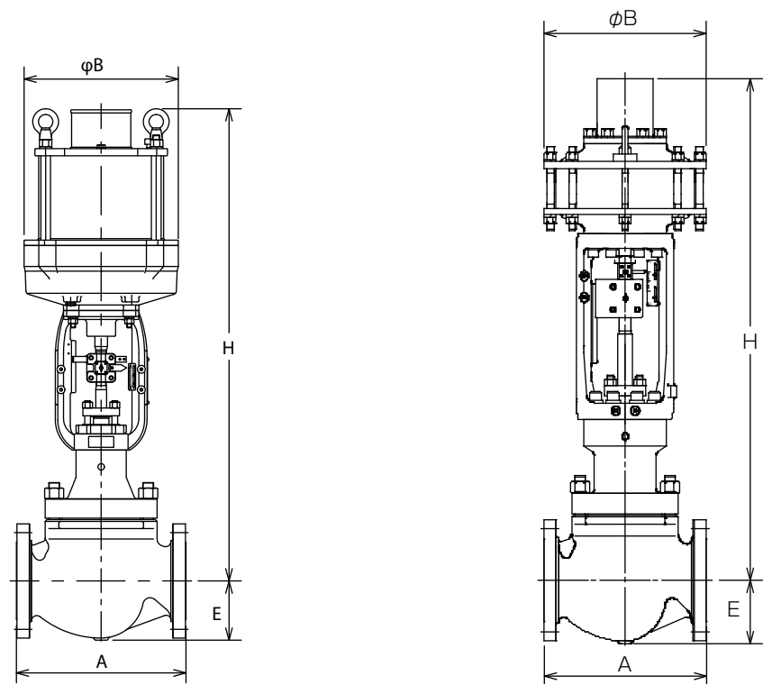
a. 适用于 PSA6/7R 执行机构 b. 适用于 DAP 执行机构
