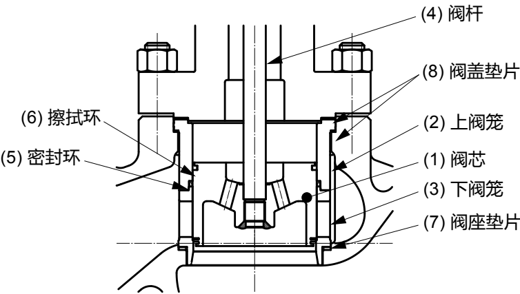
图 3. 阀内件结构图 ( 普通型 )
