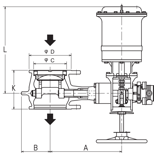
安装方式: SV0512- 400、401、800、801、070、071、080、081
