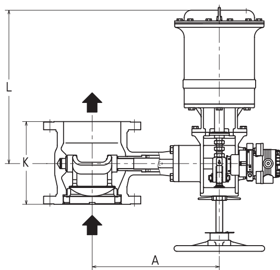
安装方式: SV0512- 200、201、600、601、030、031、040、041
