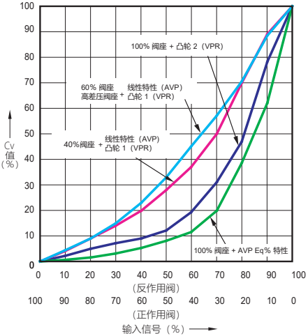
图2-3. 修正流量特性
