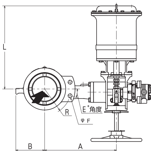
安装方式: SV0512- 100、101、500、501、010、011、020、021
