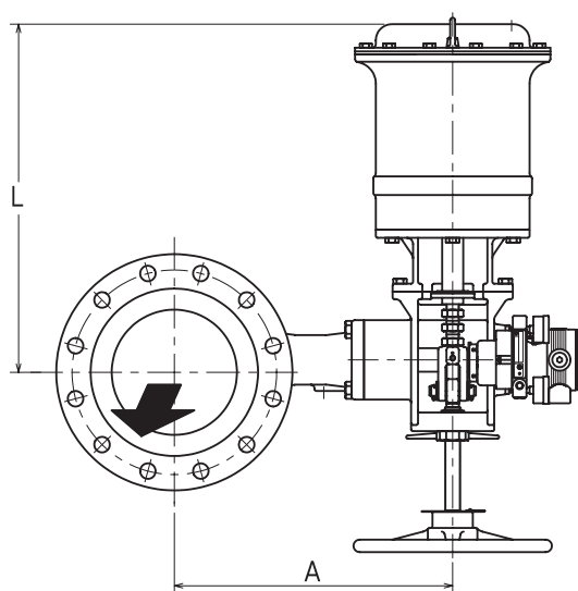
安装方式: SV0512- 300、301、700、701、050、051、060、061
