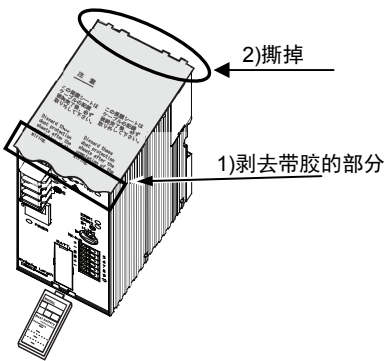
图 10 保护胶条
