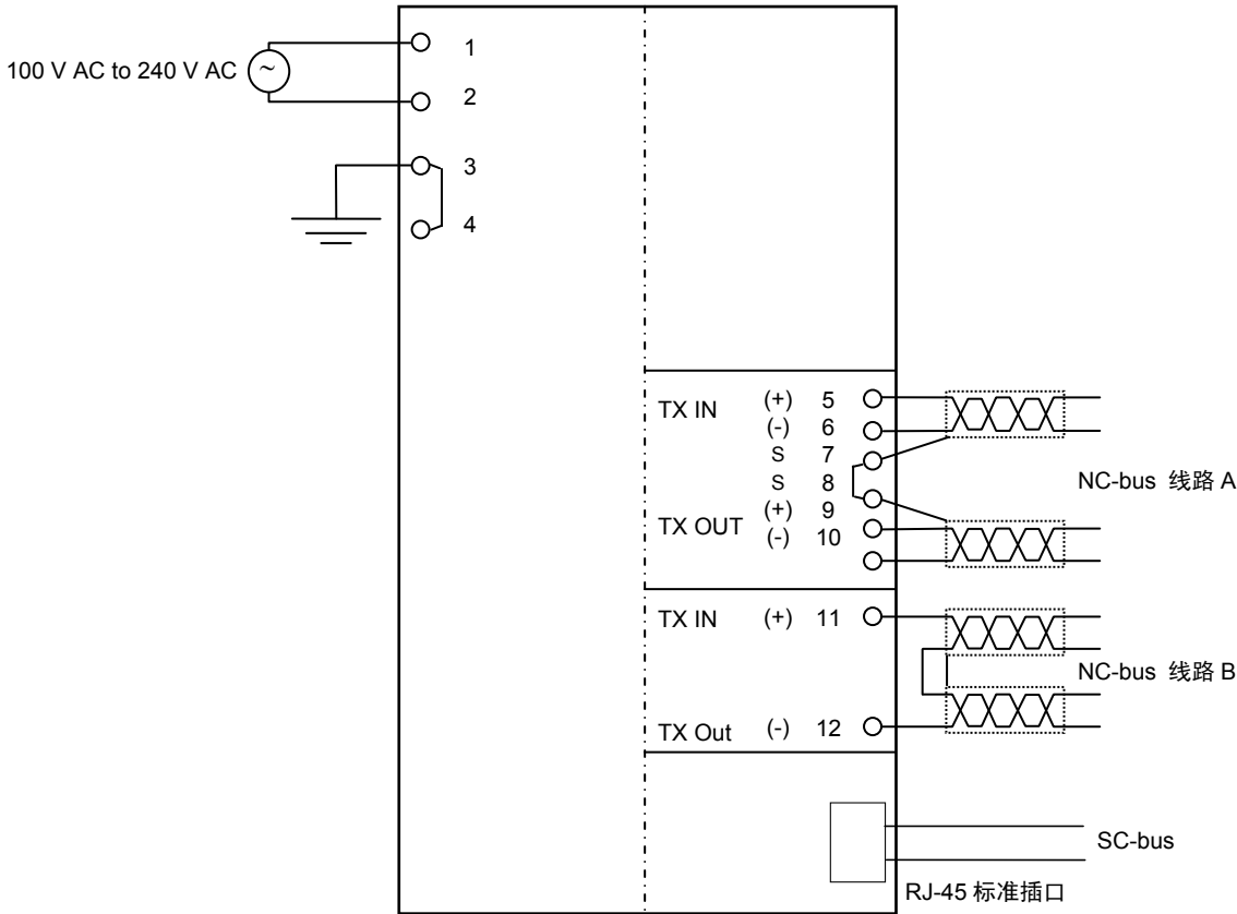
图 2 输入输出及端子配置示意图
