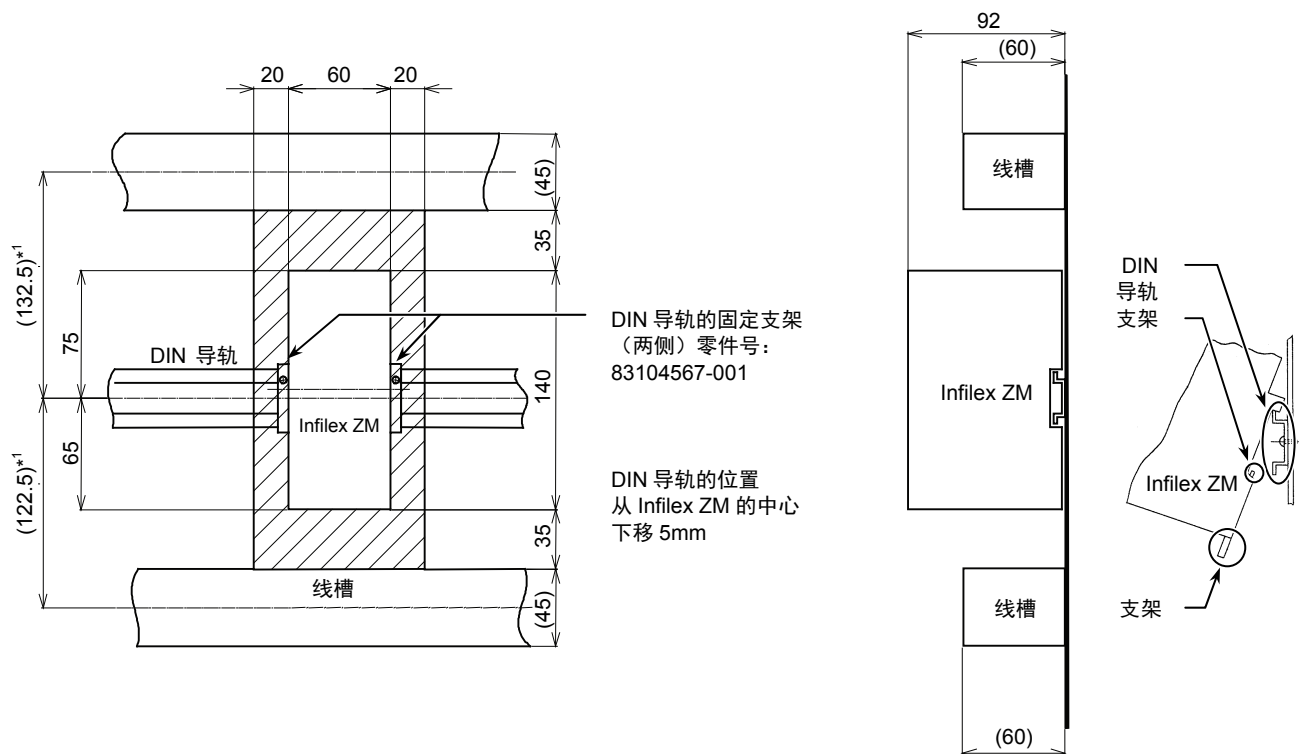
图 6 DIN 导轨的安装 (mm)
