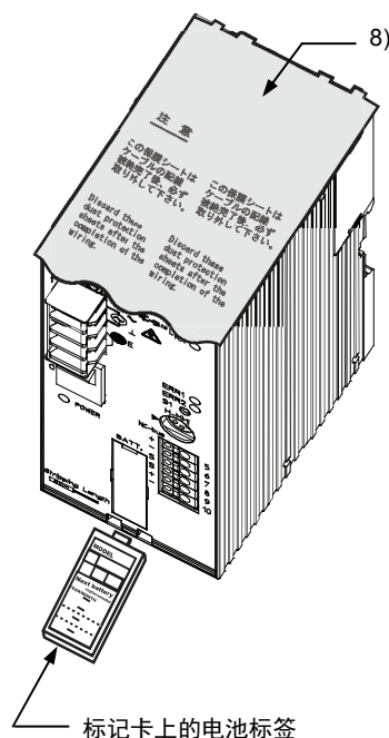
图 12 电池标签和保护用胶条
