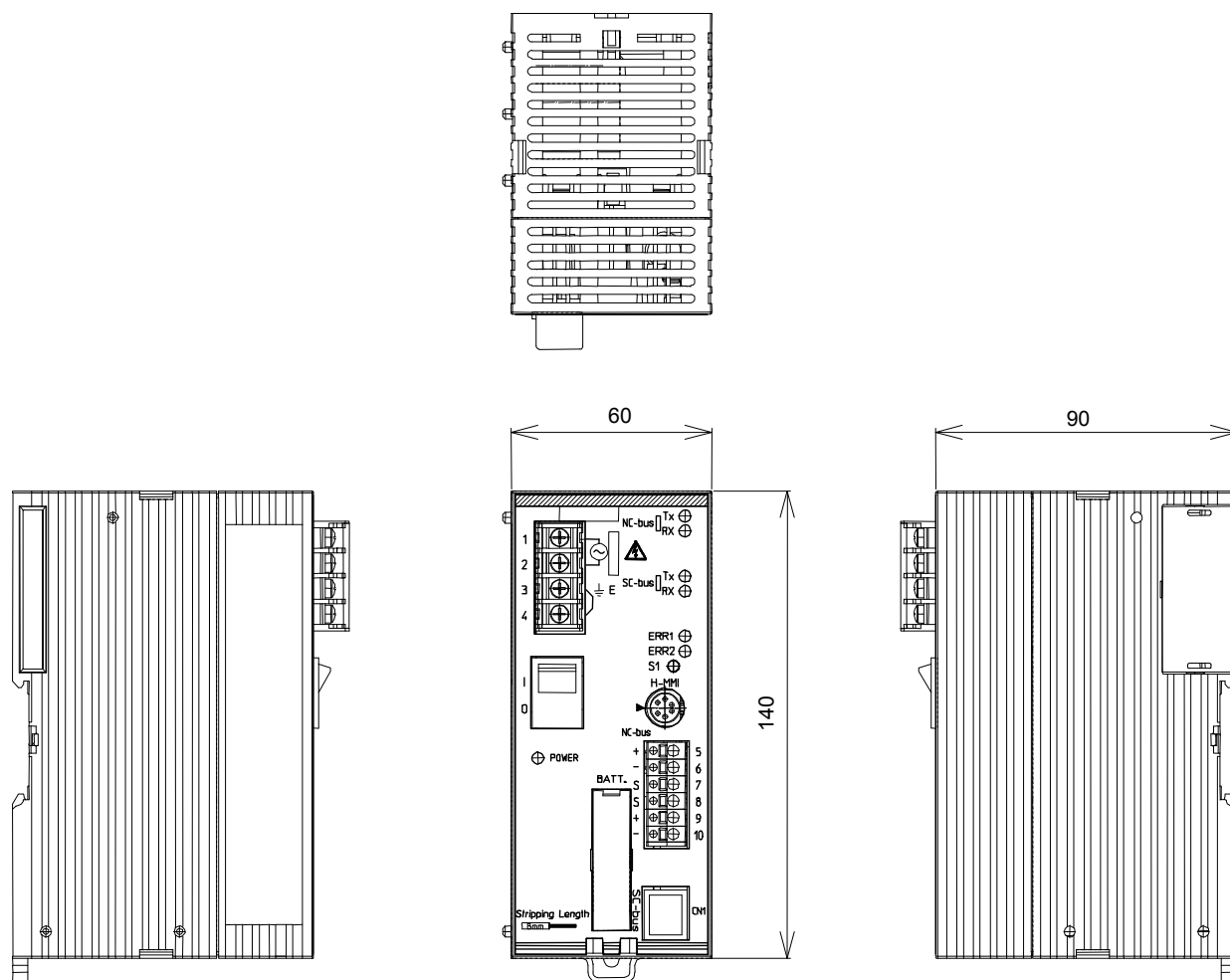
图 3 外形尺寸图 (mm)
