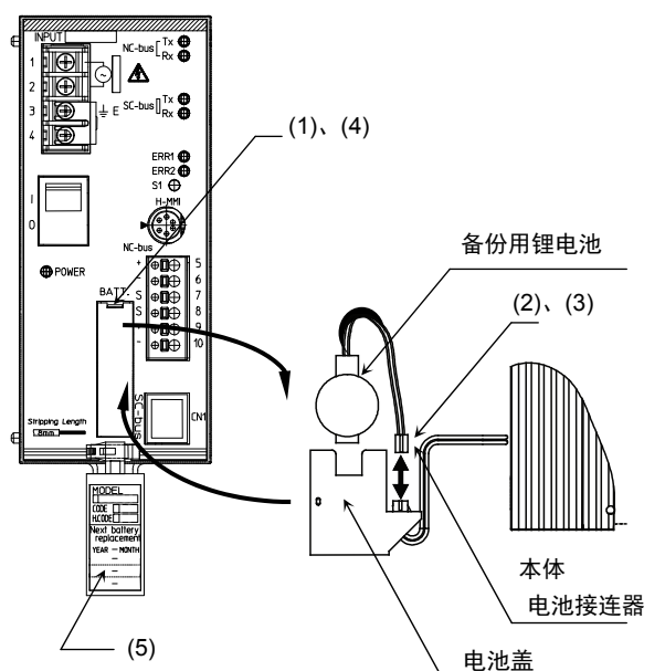
图 11 电池更换方法
