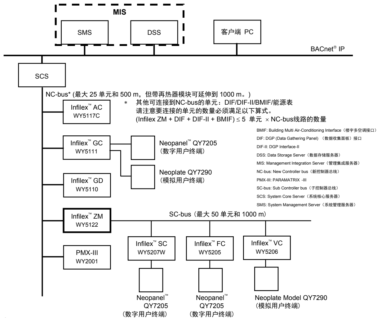
图 1. 系统配置示例
