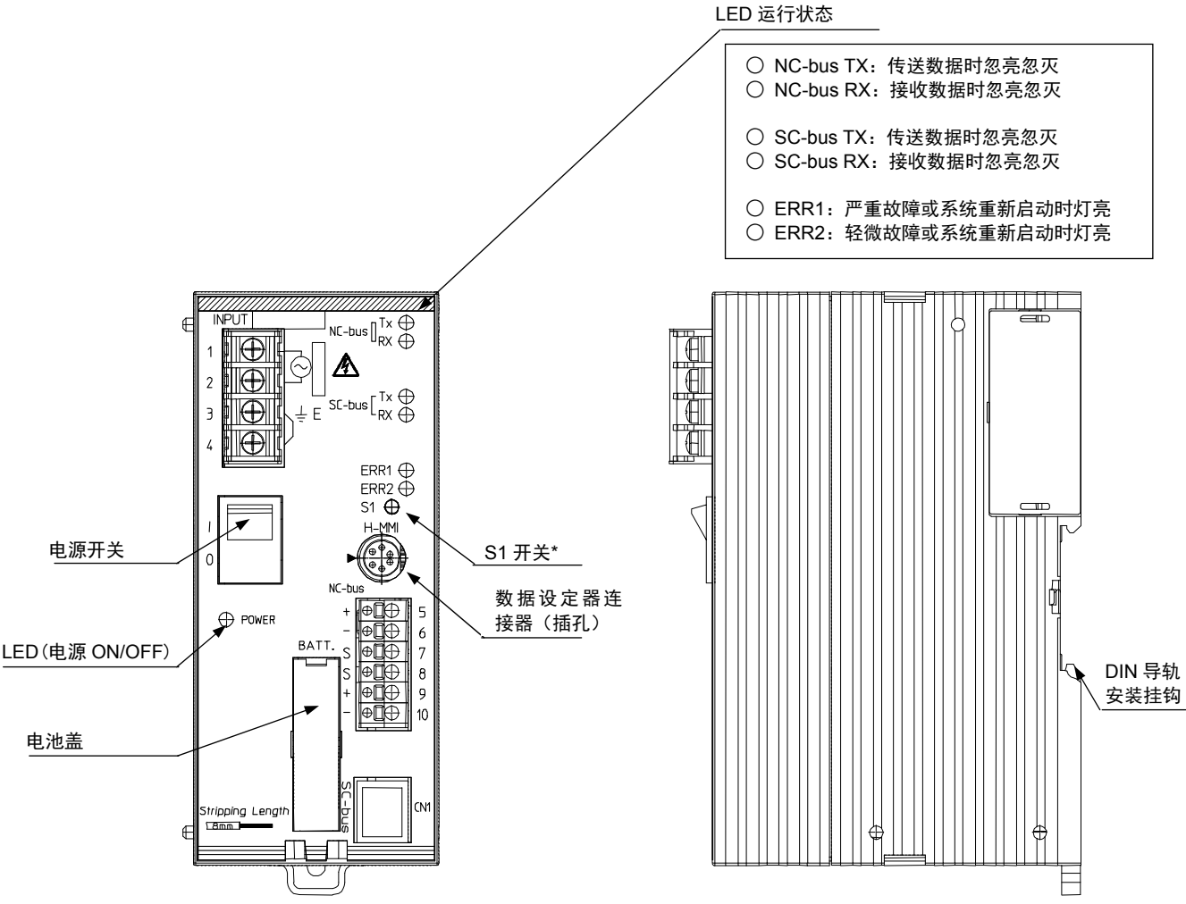
图 4 部件名称
