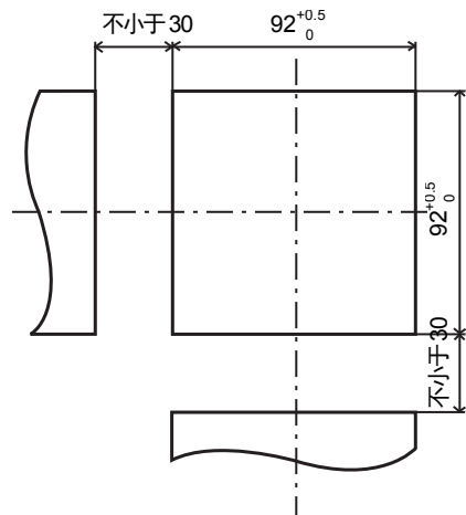
图 3 面板开孔尺寸（盘面安装型）
