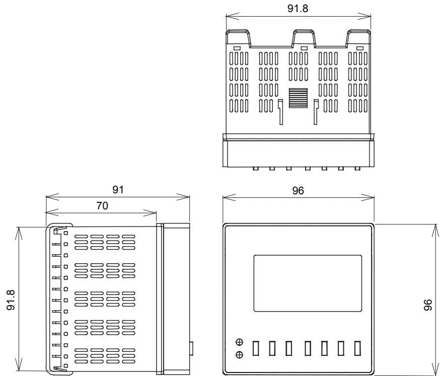
图 1 外形尺寸（盘面安装型）
