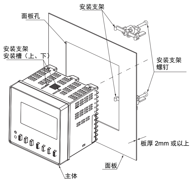
图 6 安装方法
